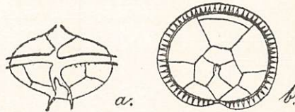
Fig. 11. Peridinium ovatum 838 1 .
