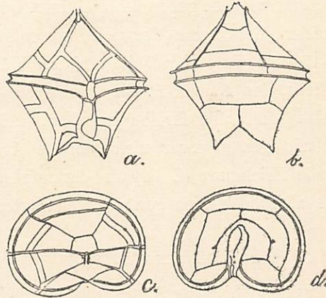
Fig. 14. Peridinium conicum 338 1 .
