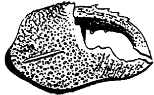
Fig. 8. Sarmatium fryatti n. sp. Chela. Magn. 1\frac{1}{2} .
